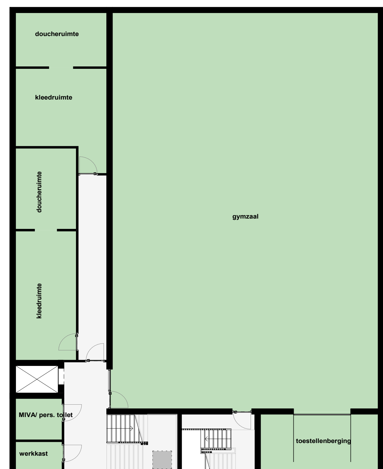
Kelder
