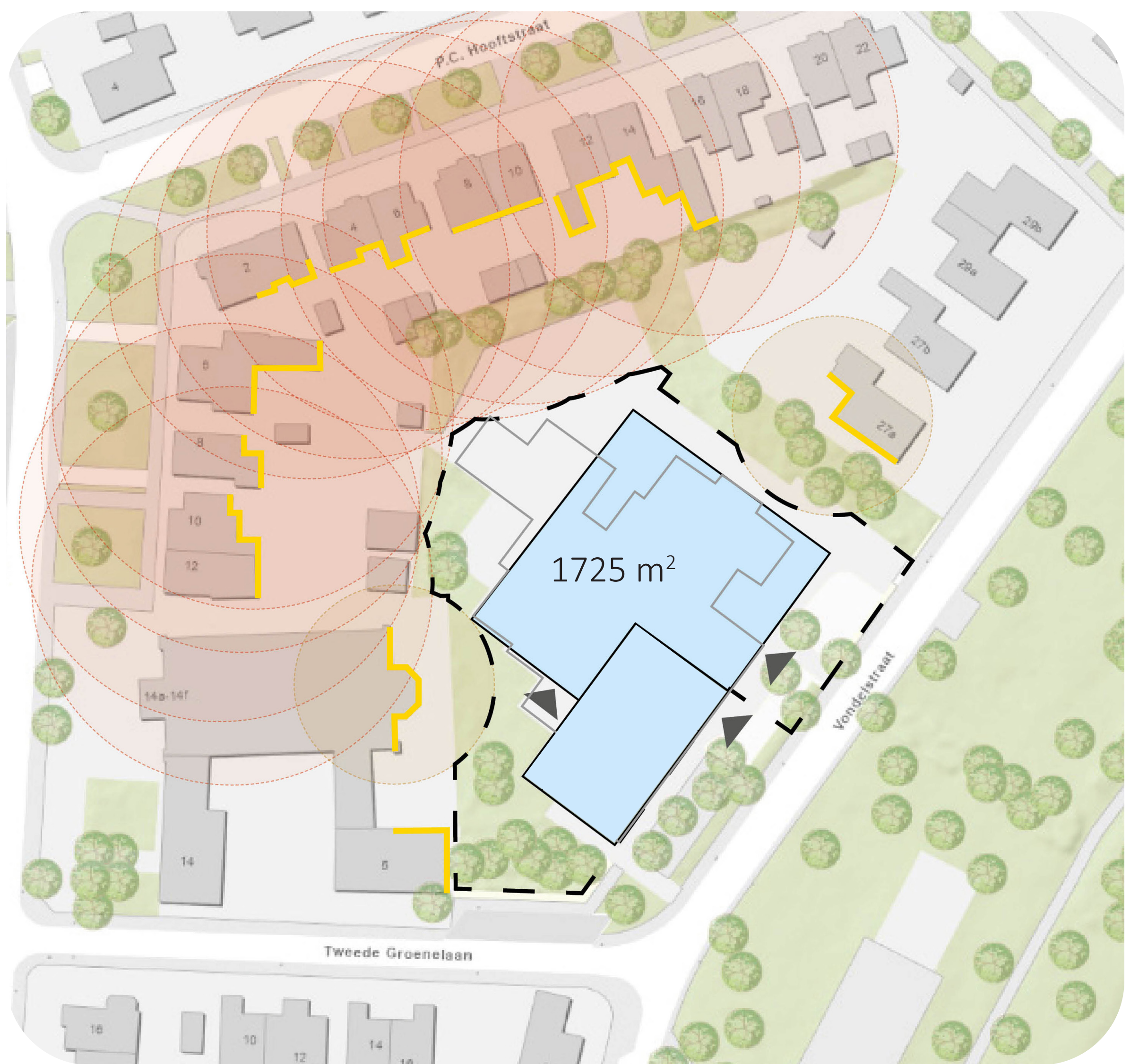
Variant gebouw met gymzaal op maaiveld
